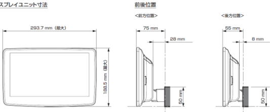
■ ディスプレイ取り付け寸法と調整可能位置 ディスプレイユニット寸法
