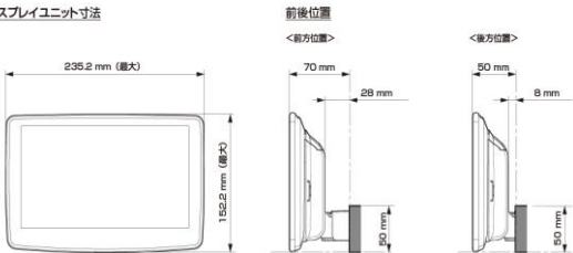
■ ディスプレイ取り付け寸法と調整可能位置 ディスプレイユニット寸法
