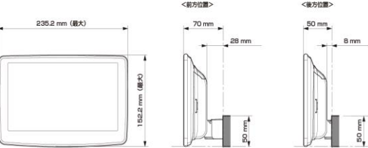
ディスプレイユニット寸法
