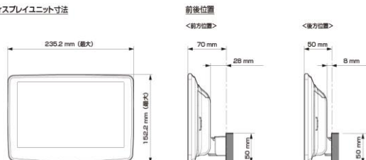
ディスプレイユニット寸法
