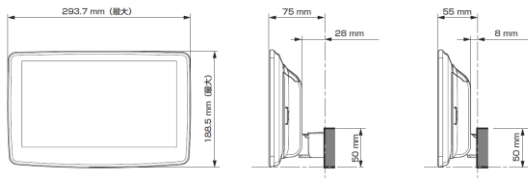
ディスプレイユニット寸法
