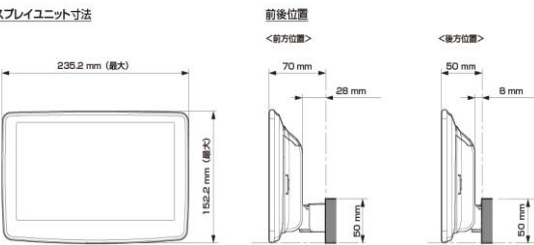
ディスプレイユニット寸法
